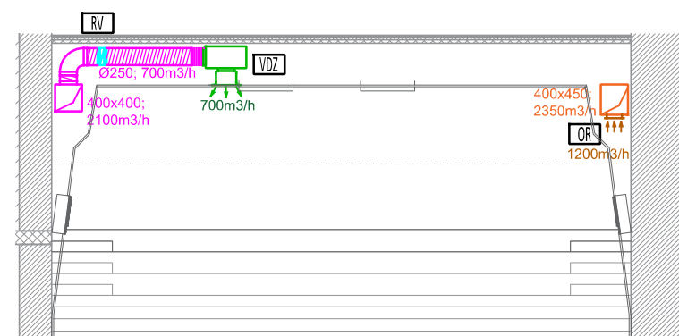
DETALJ UGRADNJE KANALA POD STROP (PRESJEK F-F)
