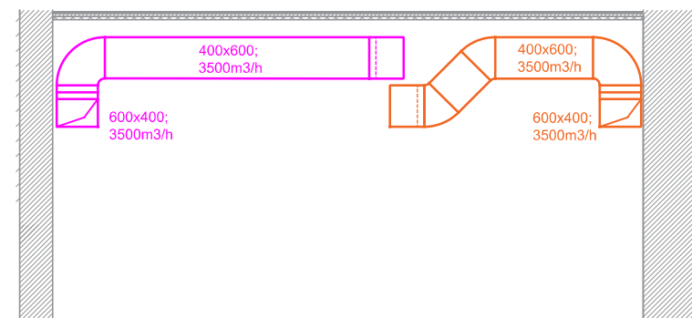
DETALJ UGRADNJE KANALA POD STROP (PRESJEK E-E)
