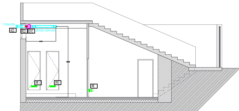
PRESJEK A-A
