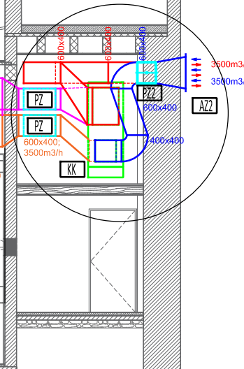
DETALJ B
