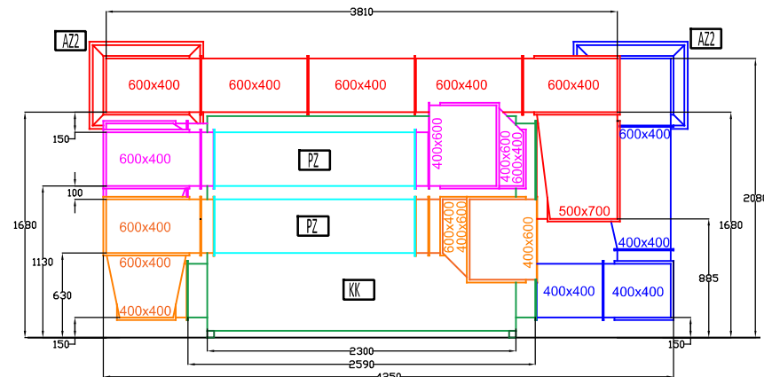
POGLED A
