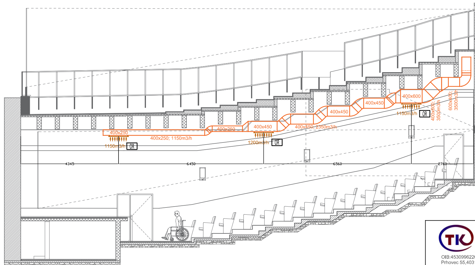
PRESJEK B-B
