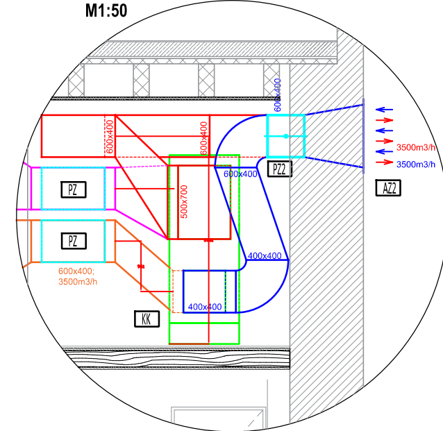
DETALJ B M1:50
