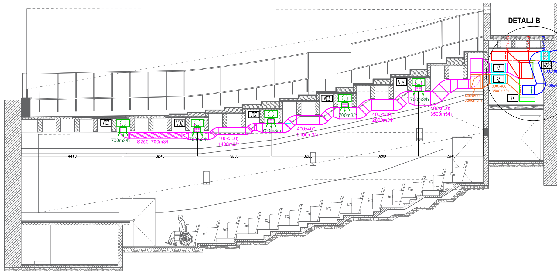
PRESJEK B-B
