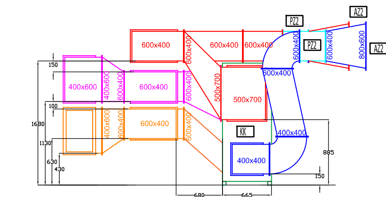
POGLED B
