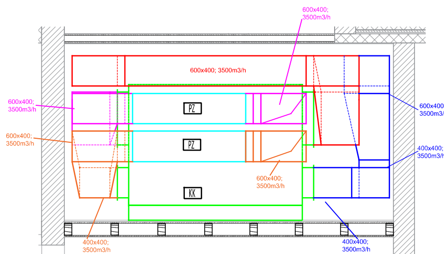
PRESJEK D-D M1:50
